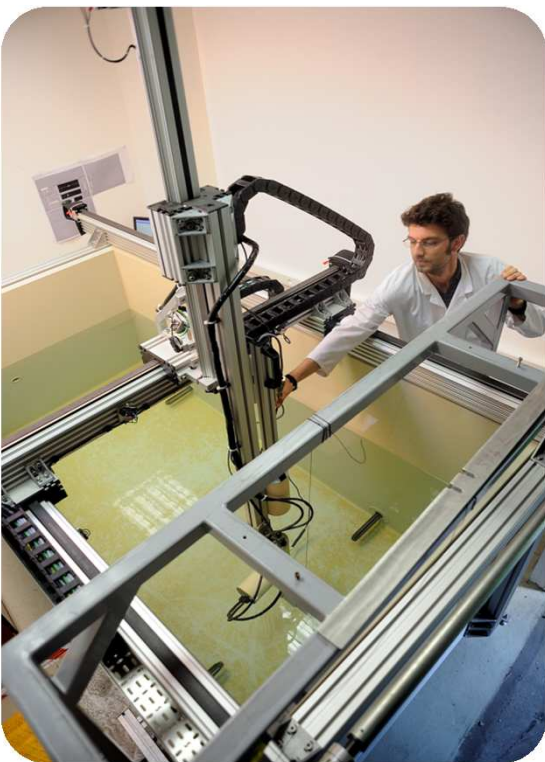
Banc d'essais VISIO (bac en eau pour expérimentations acoustiques et ultrasonores)
