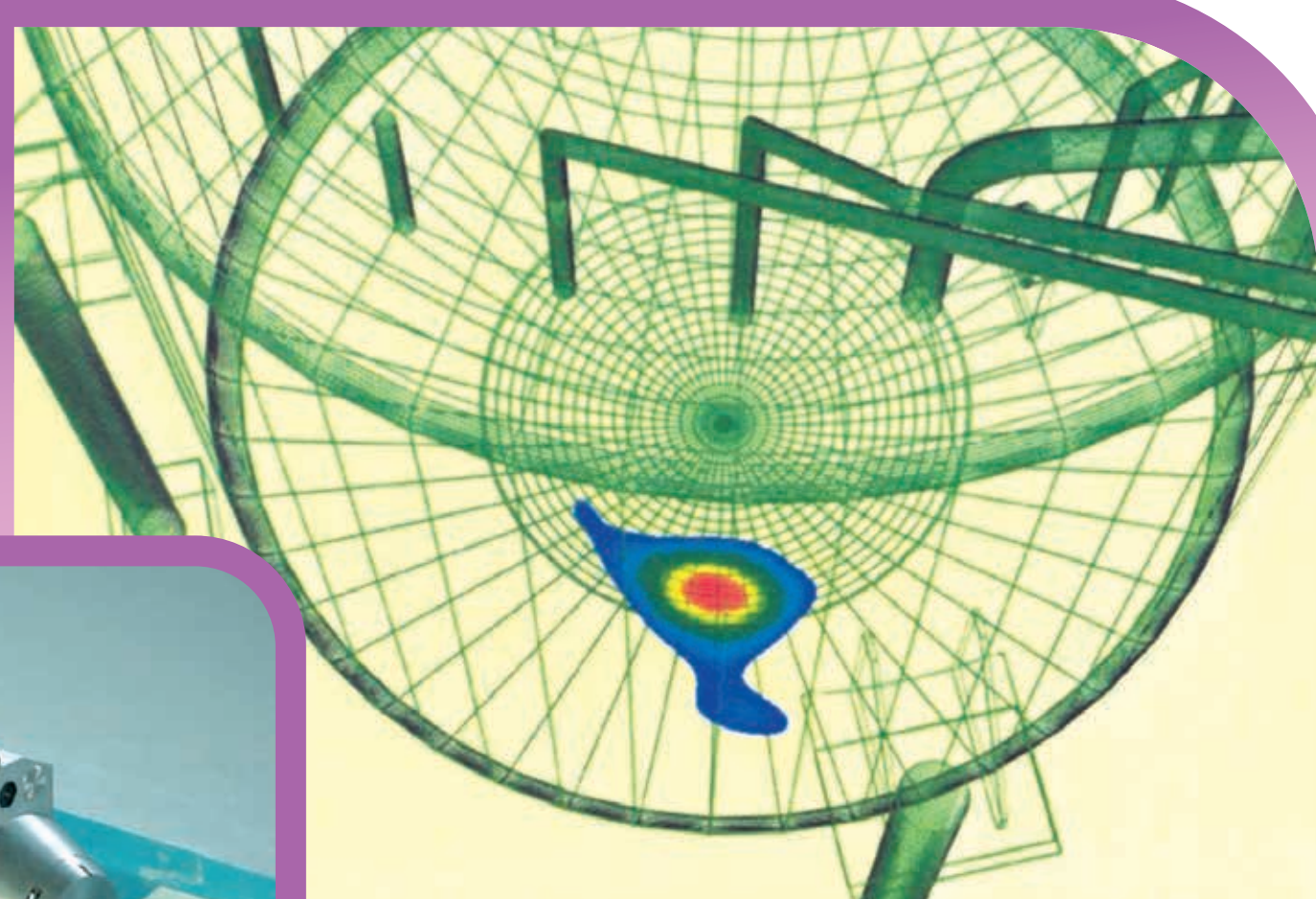
Gamma caméra
