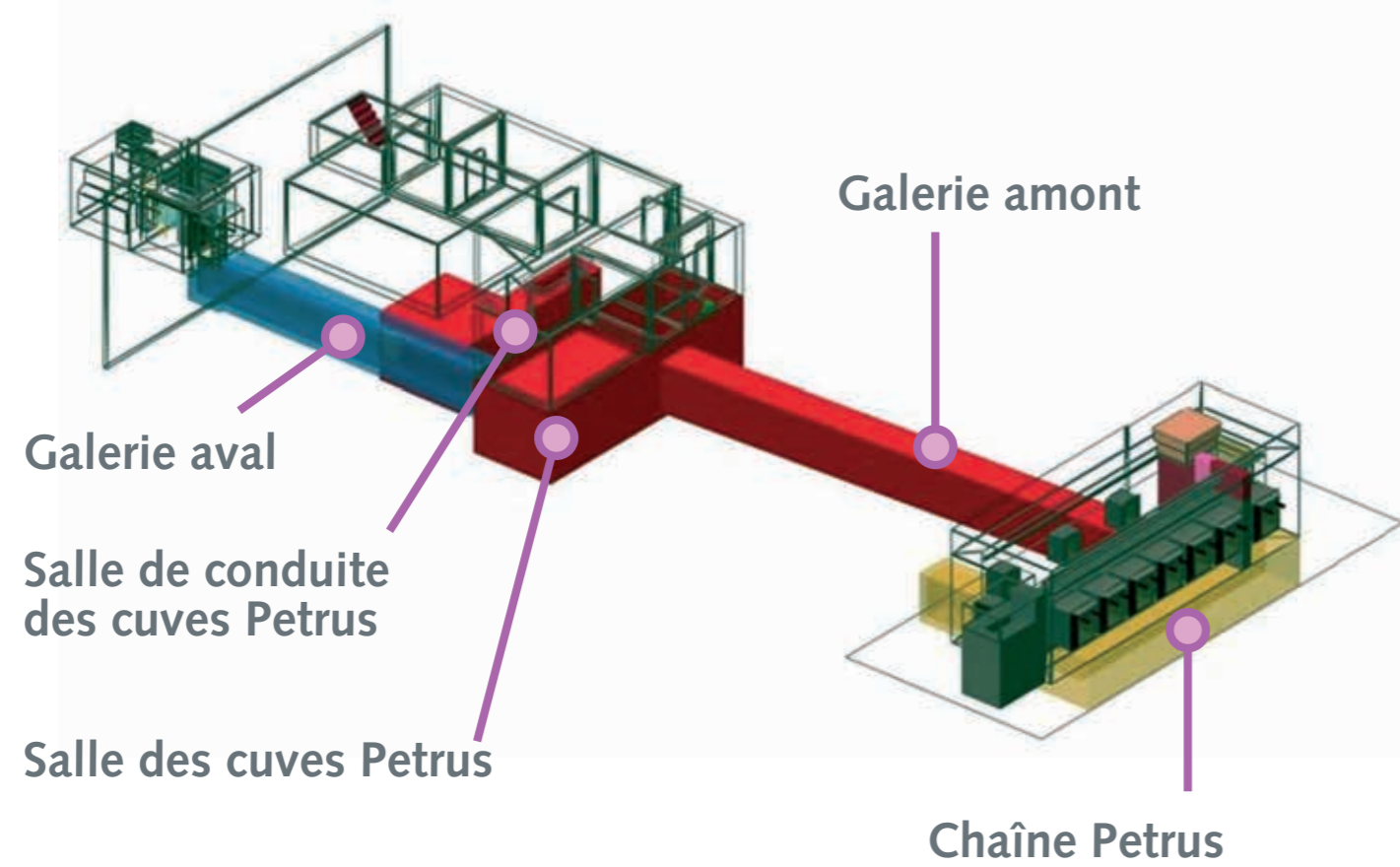
La chaîne blindée Petrus se trouve à Fontenay-aux-Roses.
