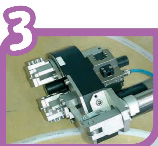
Ci-dessus : coupe-tube pneumatique développé spécialement ; ci-contre : perche de prélèvement de liquide.
