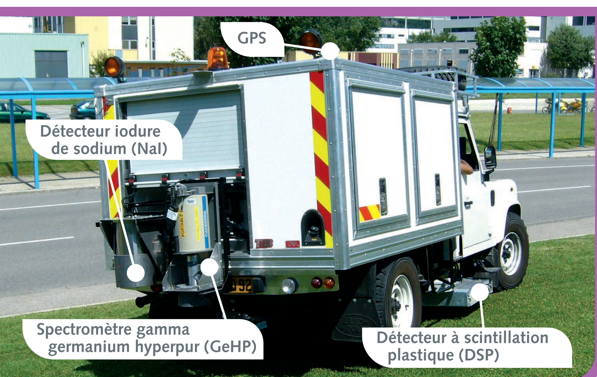
Dispositif VEGAS doté d'un régulateur de vitesse variant de 2,6 à 10 km/h, d'un GPS et de divers instruments détectant le flux de gamma émergeant du sol. Ces instruments de mesure radiologique sont positionnés à des hauteurs différentes (de 20 à 70 cm du sol) afin de différencier le flux de gamma environnant de celui, recherché, émergeant du sol. ©CEA
