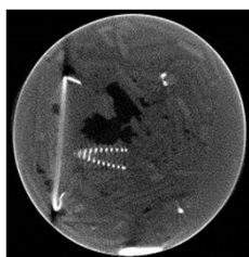
Imagerie haute énergie avec MINILINATRON : Expertise de colis de bitume sur le site de BELGOPROCESS
